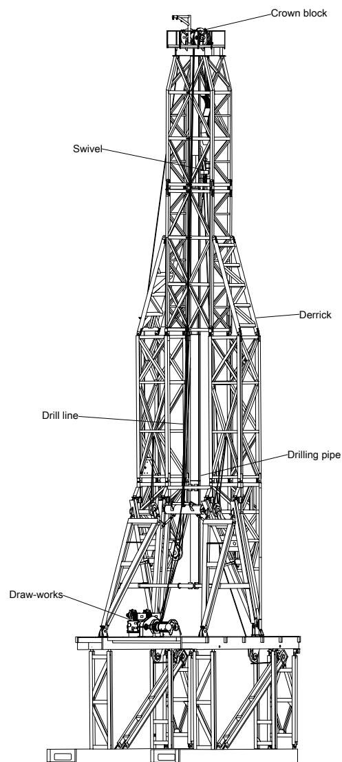
Abbildung 1: Bohrturm-Schema
